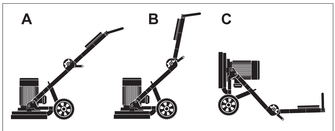
Arbeitspositionen
