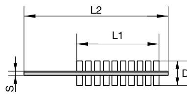
Dimensions brosses cylindriques
