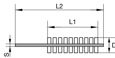
Afmetingen buisborstel
